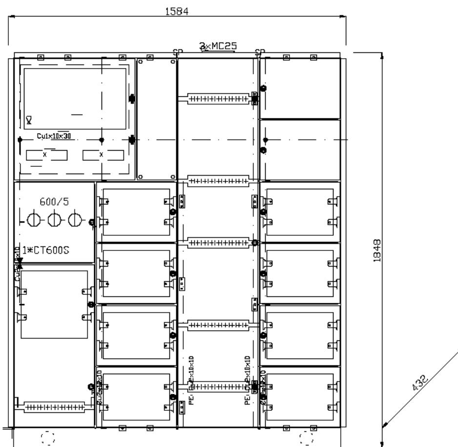
Tegning af den nye hovedtavle i forsamlingshuset.
